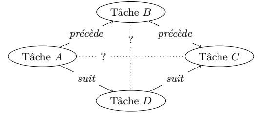
FIGURE 1 – Un réseau de contraintes temporelles simplifié, où ? désigne la disjonction de toutes les relations de base ; la contrainte entre les tâches B et D (et, de manière équivalente, A et C) n'est pas réparable, mais on peut remplacer ? par le conjonction ' \text{précède} \wedge \text{suit} ' et atteindre la paracoherence.
