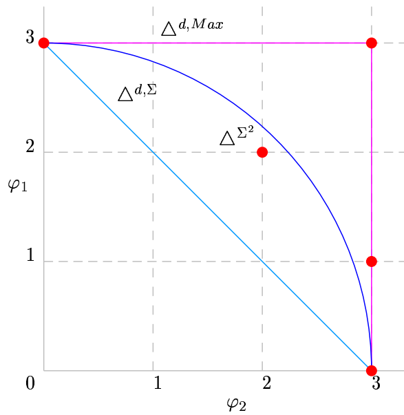
FIG. 7.1 – Fusion de deux bases de connaissance
