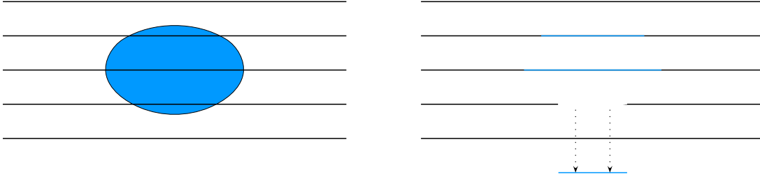
FIG. 2.2 – Révision naturelle
