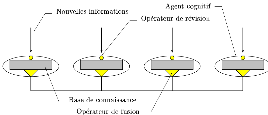
FIG. 9.1 – Système coopératif
