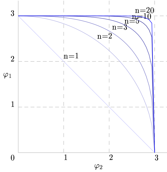
FIG. 7.2 – La famille \Delta^{d,\Sigma^n}
