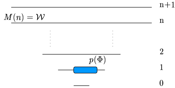
FIG. 2.3 – Modèle rangé
