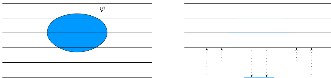
FIG. 2.6 – révision rangée
