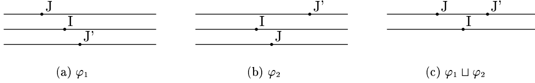
FIG. 6.2 – Arbitrage
