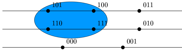
FIG. 1.7 – Information conditionnelle
