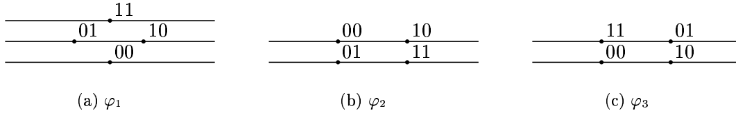
FIG. 8.3 – Pré-ordres
